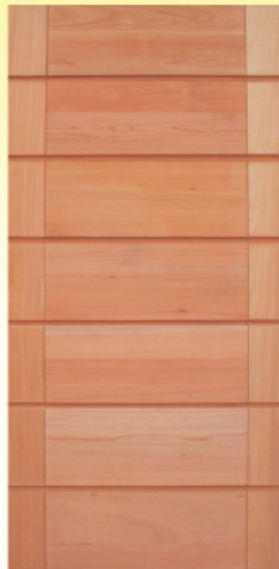
PORTA PIVOTANTE BBB-R CÓDIGO 2007 - 2,10m x 0,62m CÓDIGO 2008 - 2,10m x 0,72m CÓDIGO 2009 - 2,10m x 0,82m CÓDIGO 2010 - 2,10m x 0,92m CÓDIGO 2011 - 2,10m x 1,02m CÓDIGO 2012 - 2,10m x 1,12m CÓDIGO 2013 - 2,10m x 1,22m
